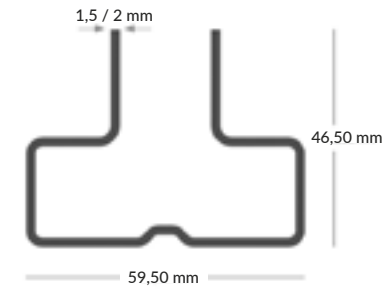
F60 MR AYAK PROFİL KESİTİ
